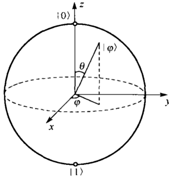
图 3.10: 布洛赫球
