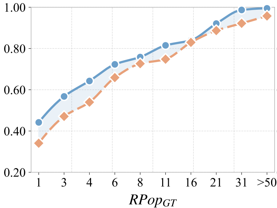
Llama-3-8B
