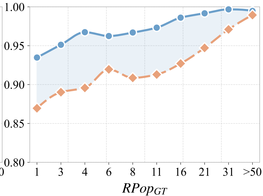
ChatGPT
