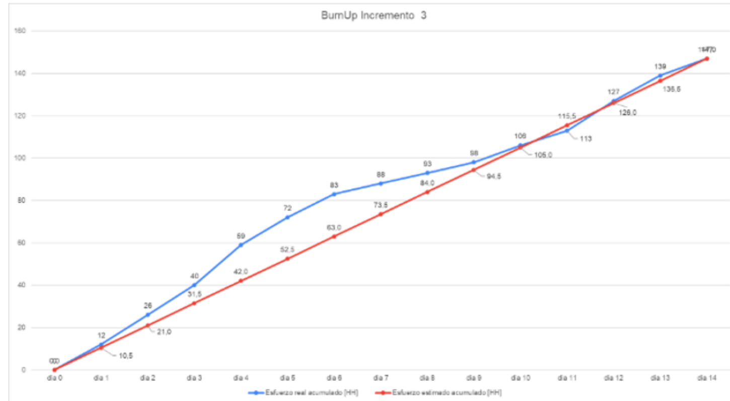
Figura 14.5 Gráfica burn-up de esfuerzos del equipo.
