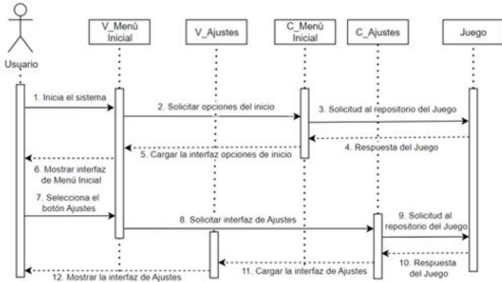
Figura 4.3: "Caso de Uso N°2, Entrando a Ajustes".
