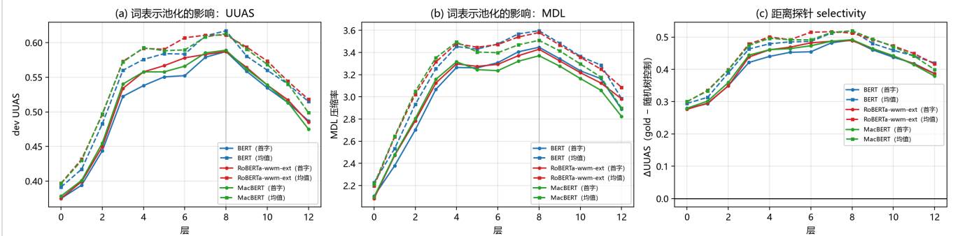
图 4 均值池化消融: 峰值层不变, 绝对值整体上移
