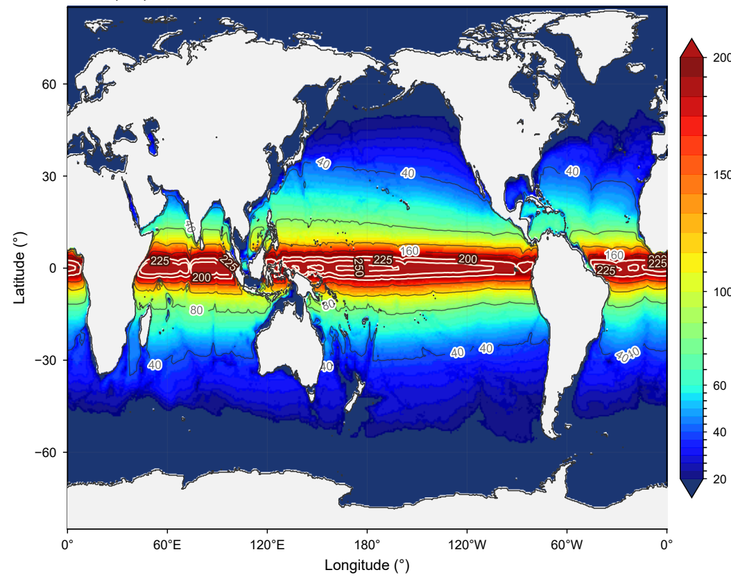
b L_d (km)
