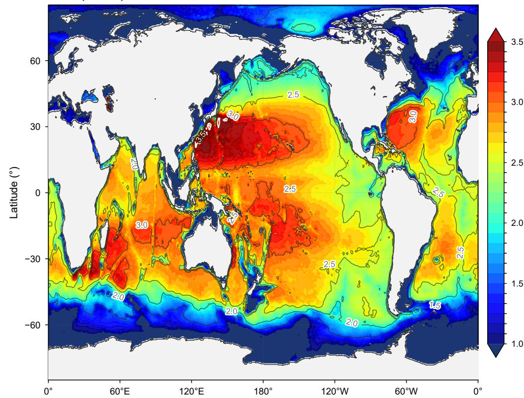
a c_1 ( \text{m s}^{-1} )
