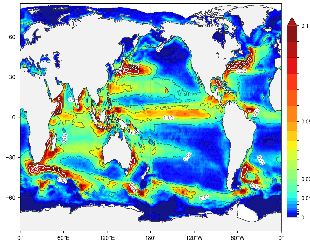
c EKE ( \text{m}^2 \text{s}^{-2} )
