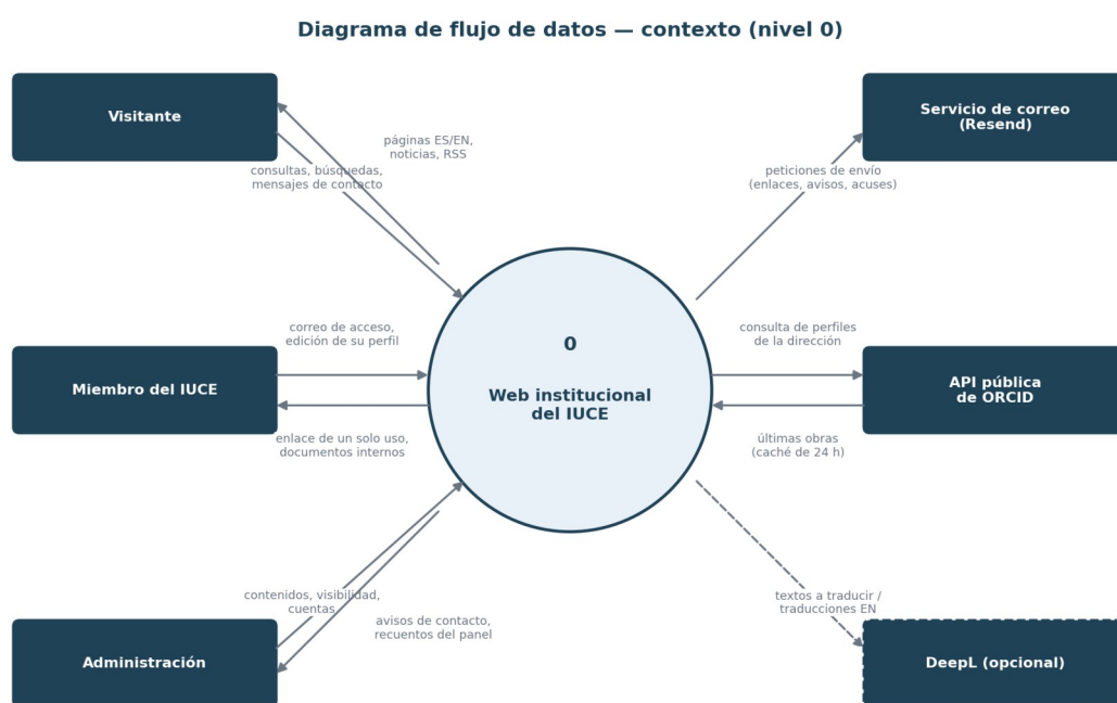
Figura 3. Diagrama de flujo de datos de contexto (nivel 0).
