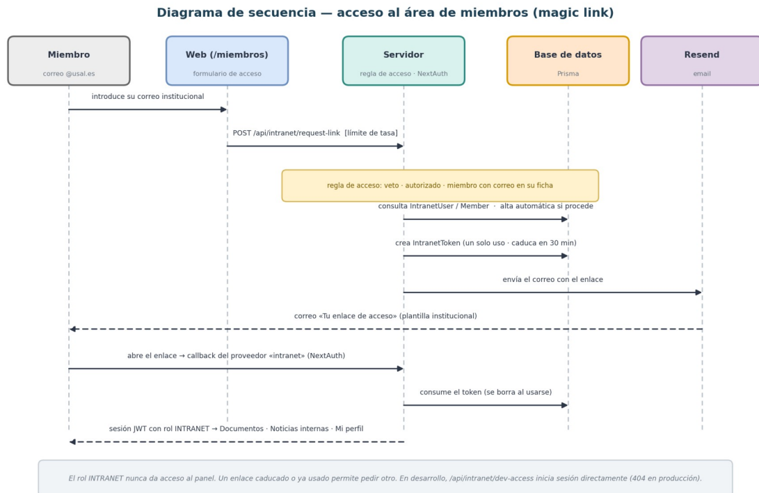
Figura 5. Diagrama de secuencia del acceso al área de miembros.
