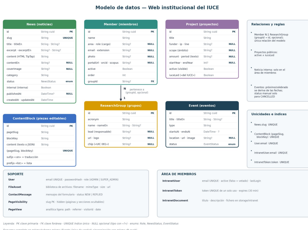
Figura 4. Modelo de datos: entidades y campos, relación Member–ResearchGroup, reglas y unicidades.
