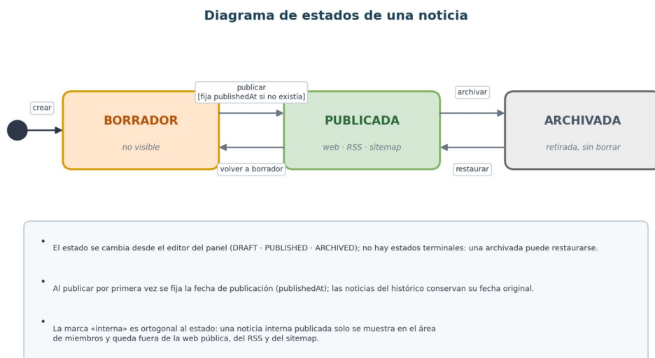
Figura 6. Diagrama de estados de una noticia (transiciones y reglas).
