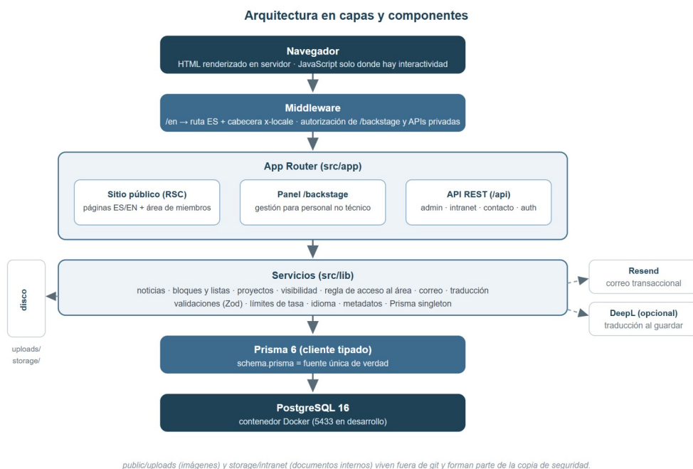
Figura 5. Arquitectura en capas y componentes del sistema.
