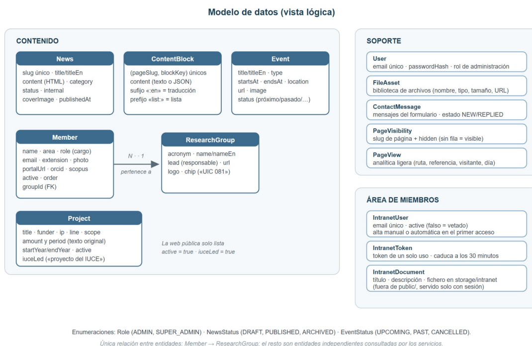
Figura 2. Modelo de datos (vista lógica): entidades, campos principales y relación Member–ResearchGroup.
