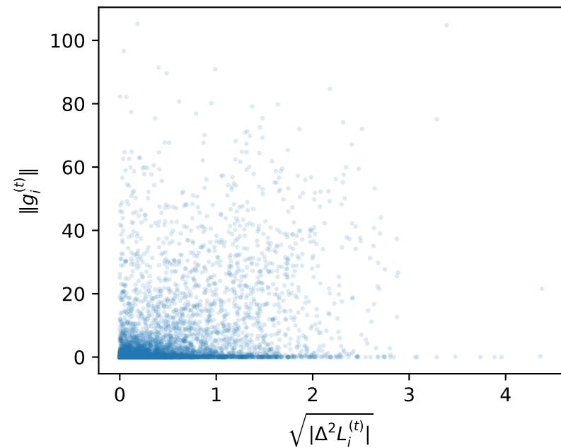
Adam (corr=0.478)
