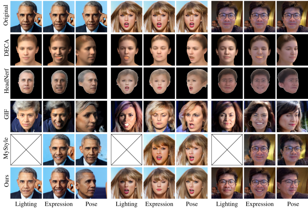
図 2.12: DECA と他モデルとの比較結果 [22].
