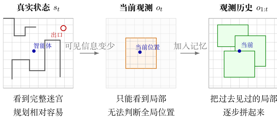
图 1: 从完全观测到不完全观测，再到利用观测历史补全信息。关键变化不在环境本身，而在智能体手里可用于决策的信息量。
