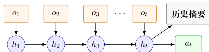
图 2: RNN 顺序读取观测历史 o_1, \dots, o_t ，并把它们压缩成当前隐藏状态 h_t 。动作 a_t 不是只依赖最新观测，而是依赖这个“历史摘要”。
