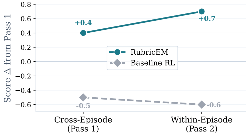
(d) Inference-Time Experience Reuse
