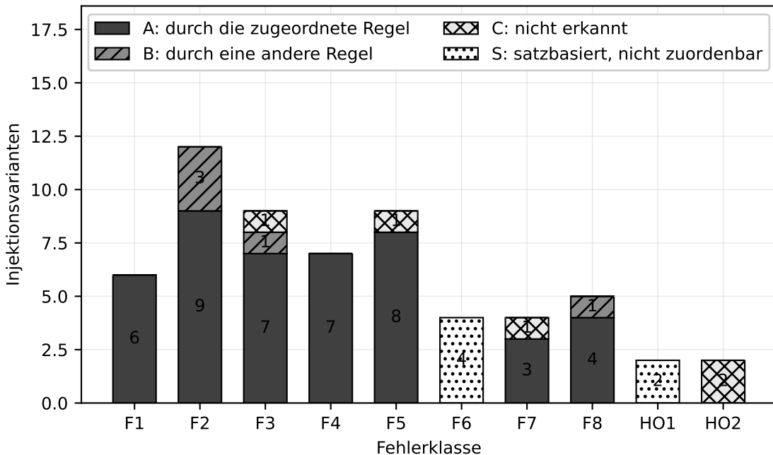
Trefferkategorien je Fehlerklasse (Teilversuch T6)
