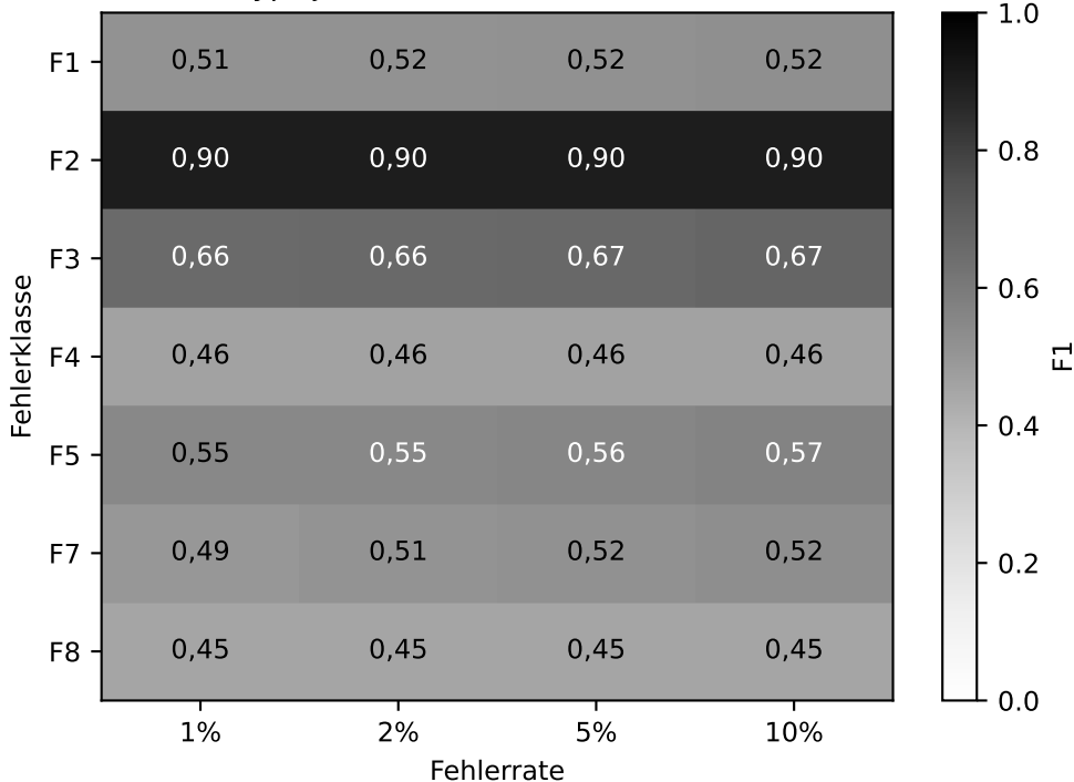
F1 des Prototyps je Fehlerklasse und Fehlerrate (Zellebene)
