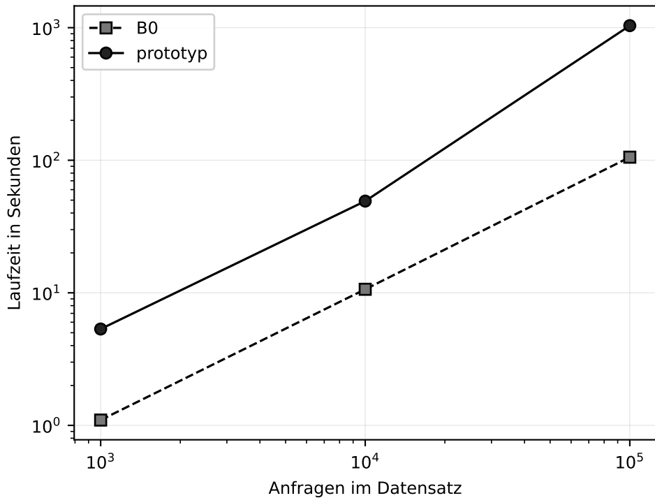
Laufzeit ueber Datensatzgroesse (Teilversuch T4)
