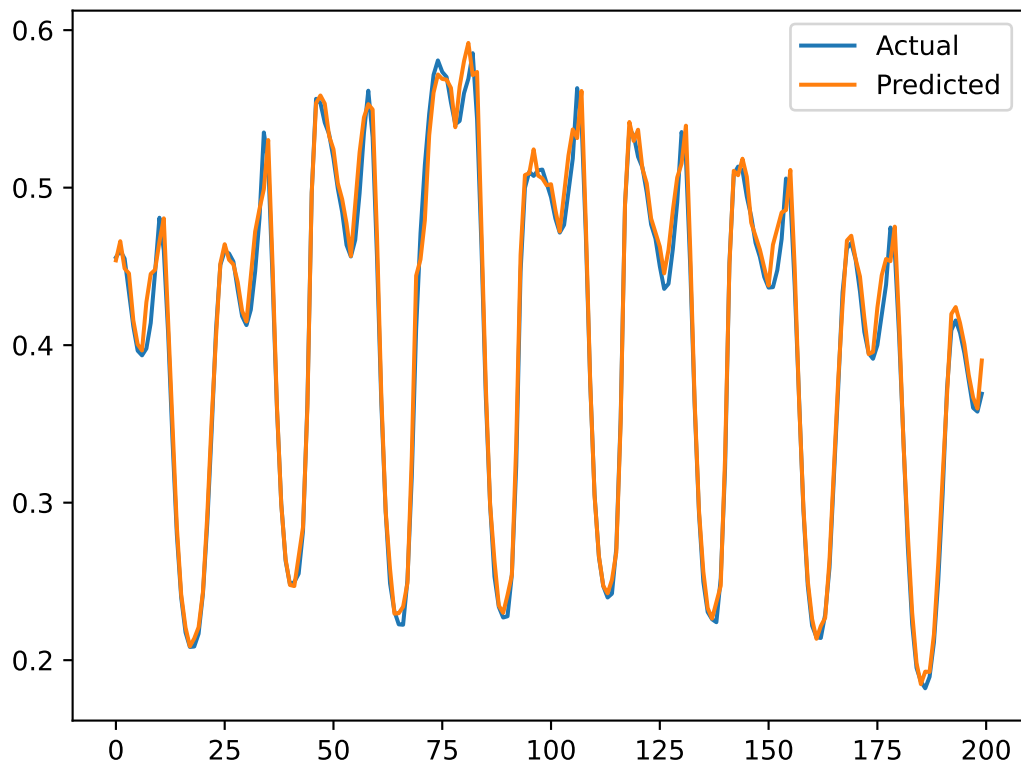
RQ1: Load Forecast vs Actual
