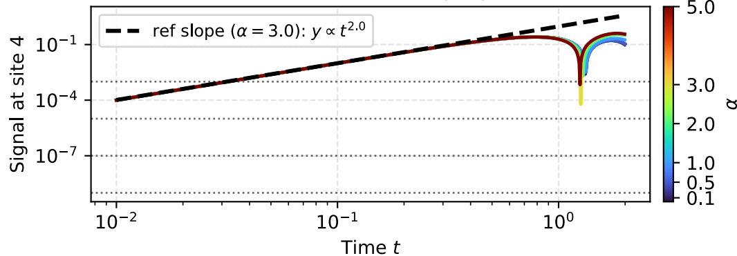
N = 50, J_x = 0.5
