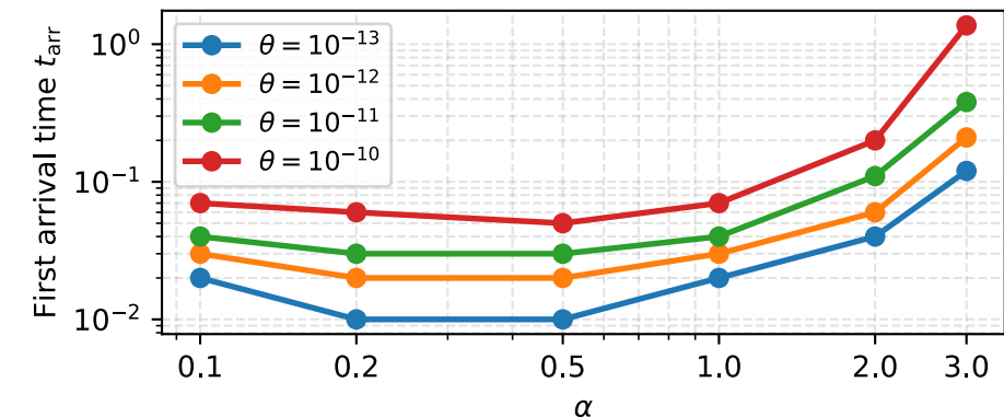
N = 50, J_x = 0.5
