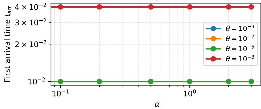
N = 50, J_x = 0.5
