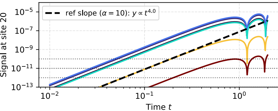
N = 50, J_x = 0.5
