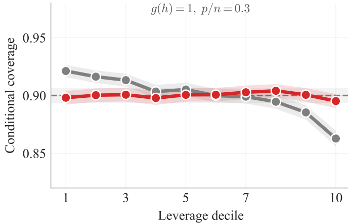
Homoscedastic
