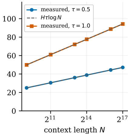
(a) LSE normalisation
