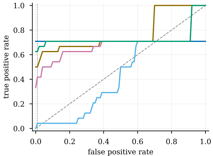
mistral-7b, N = 4096 , layer 16
