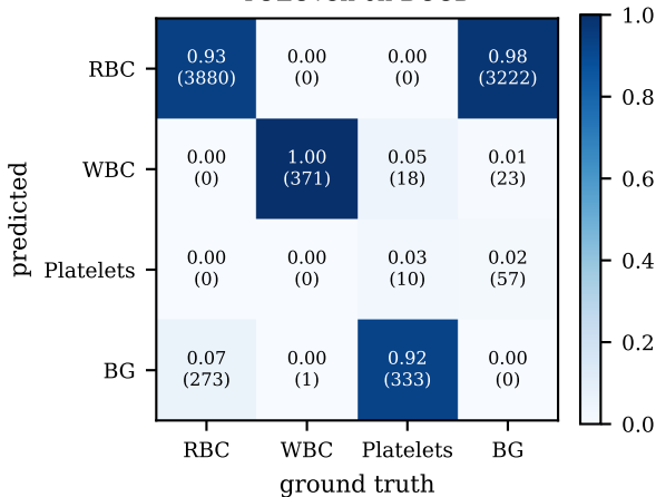
YOLOv8n on BCCD
