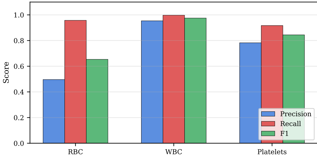
Per-class Precision / Recall / F1 (BCCD test set)
