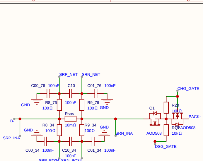
电流采样回路
