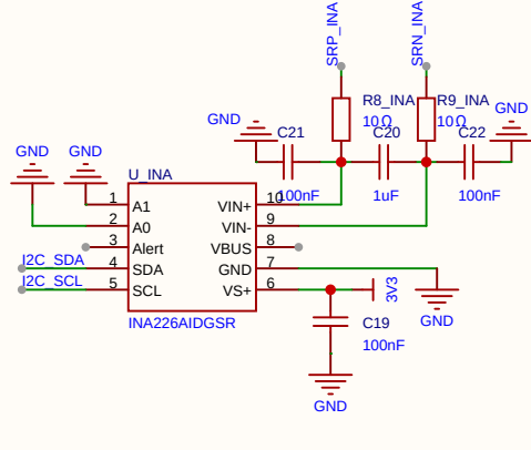
INA226 高精度电流测量
