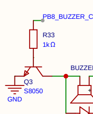
蜂鸣器
