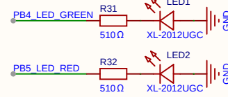
LED指示
