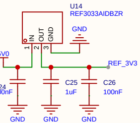
REF3033 提供基准电压
