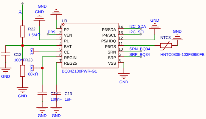
BQ34Z100PWR-G1 阻抗追踪 容量计算
