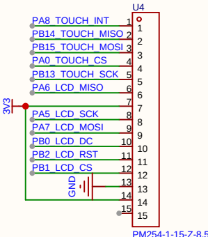
LCD排母
