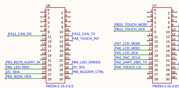
G474RET主控排母
