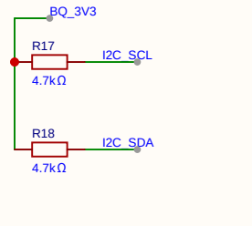
IIC总线
