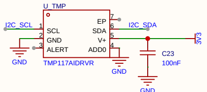
TMP117 高精度温度测量
