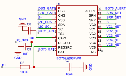
BQ76920 单体均衡 电池电压采集
