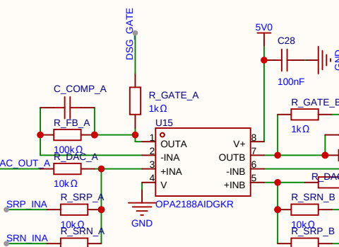
OPA2188
