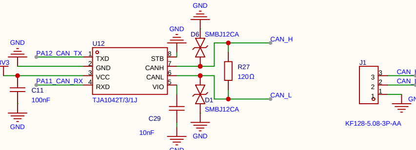
CAN收发器
