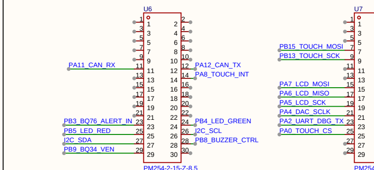
G474RET主控排母
