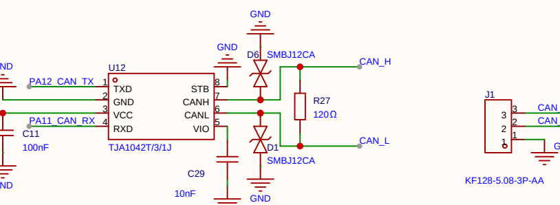
CAN收发器
