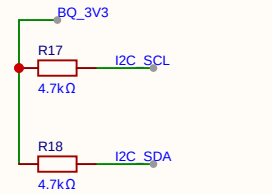
IIC总线
