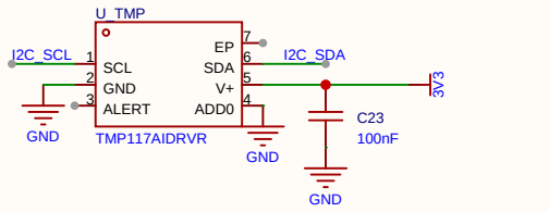
TMP117 高精度温度测量
