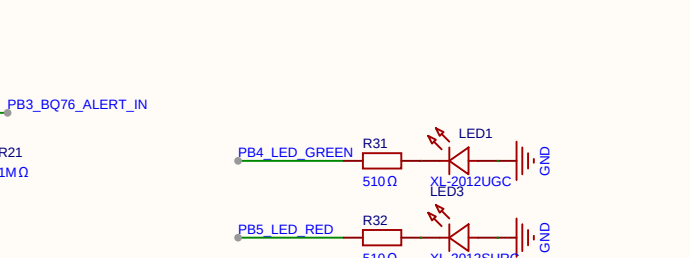
LED指示
