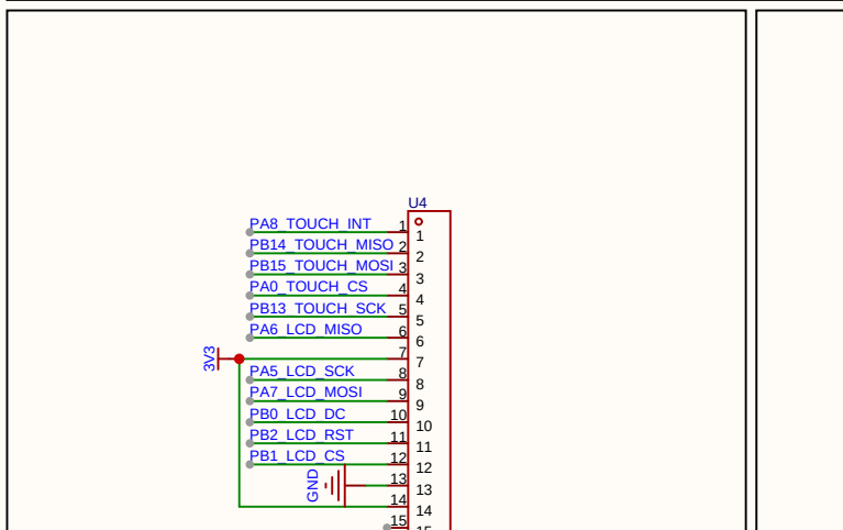
G474RET主控排母
