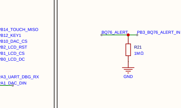
BQ_ALERT中断
