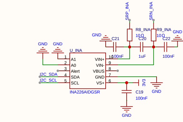
INA226 高精度电流测量
