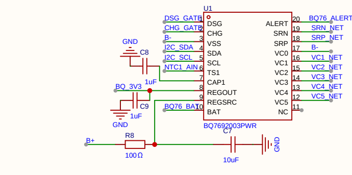
BQ76920 单体均衡 电池电压采集
