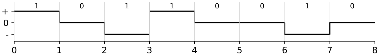
Bipolar AMI
