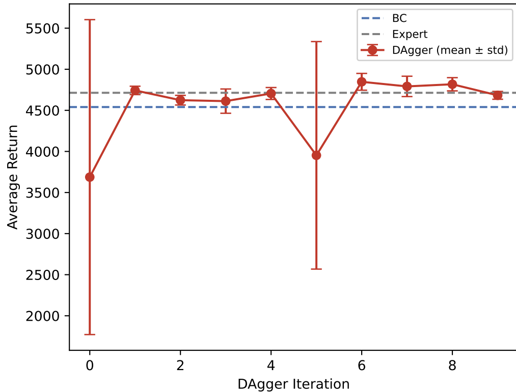
Ant-v2
