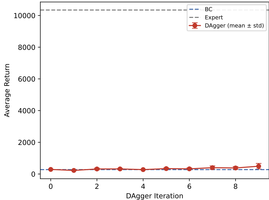
Humanoid-v2
