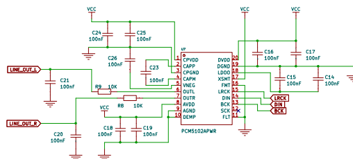
DAC
