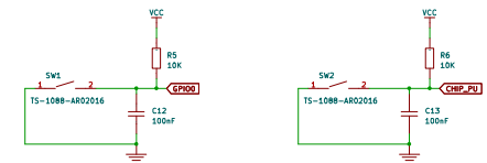
Buttons
