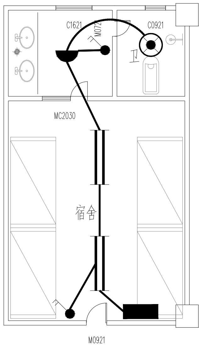
宿舍照明布置大样图
