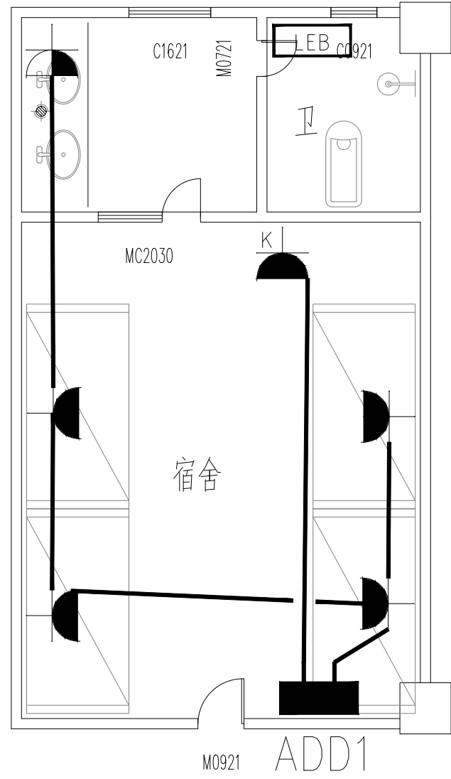
宿舍插座布置大样图
