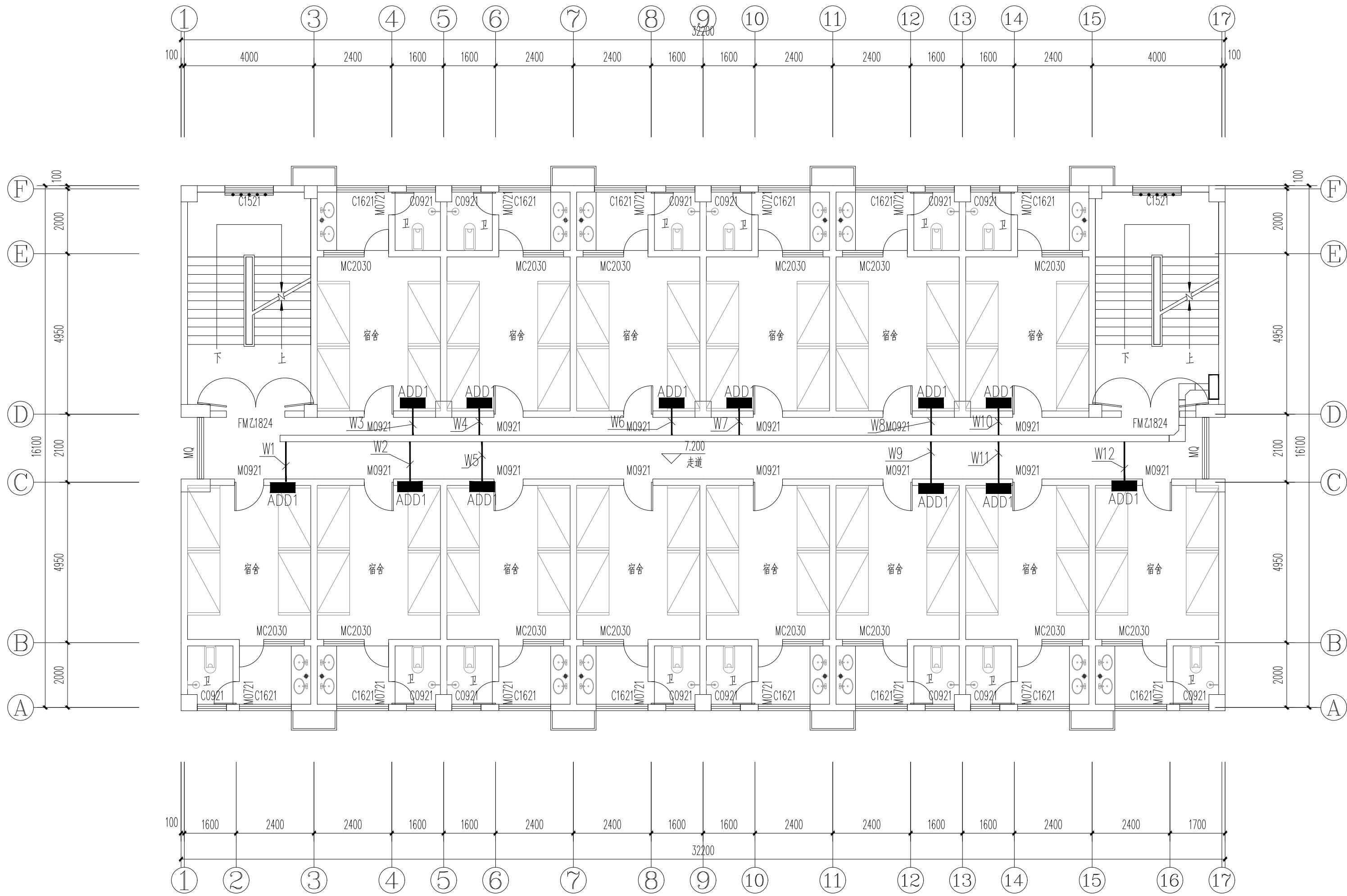
三层平面图 1:100
