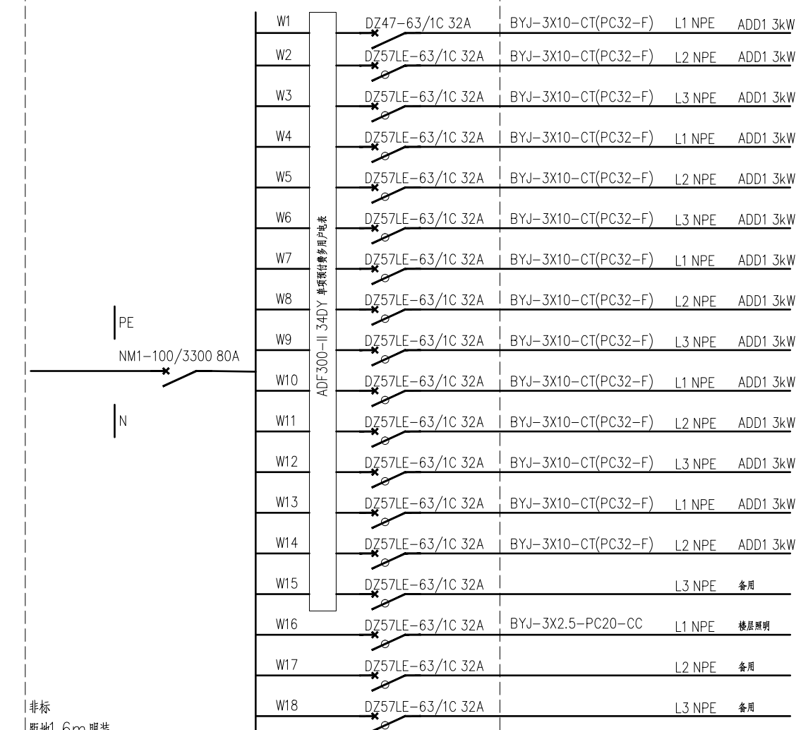
2AL1系统图
