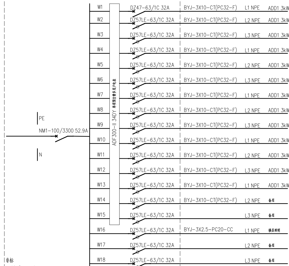
3AL1系统图
