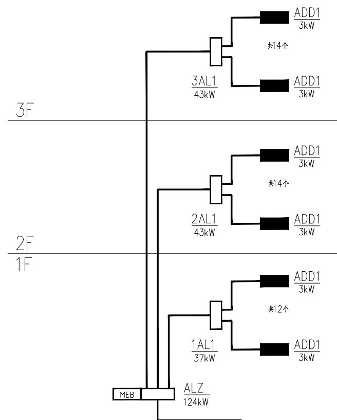
竖向配电系统图
