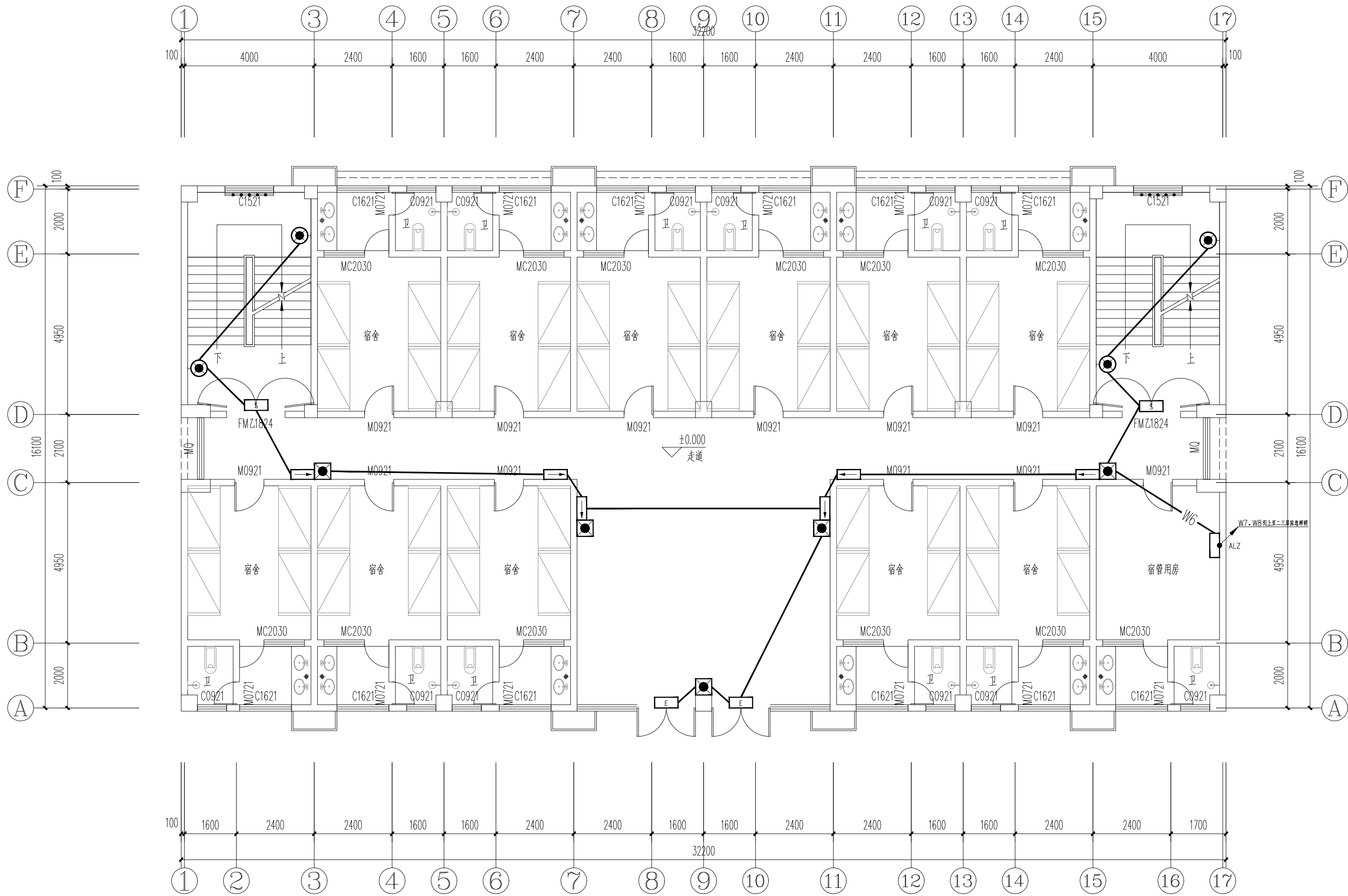
一层平面图 1:100
