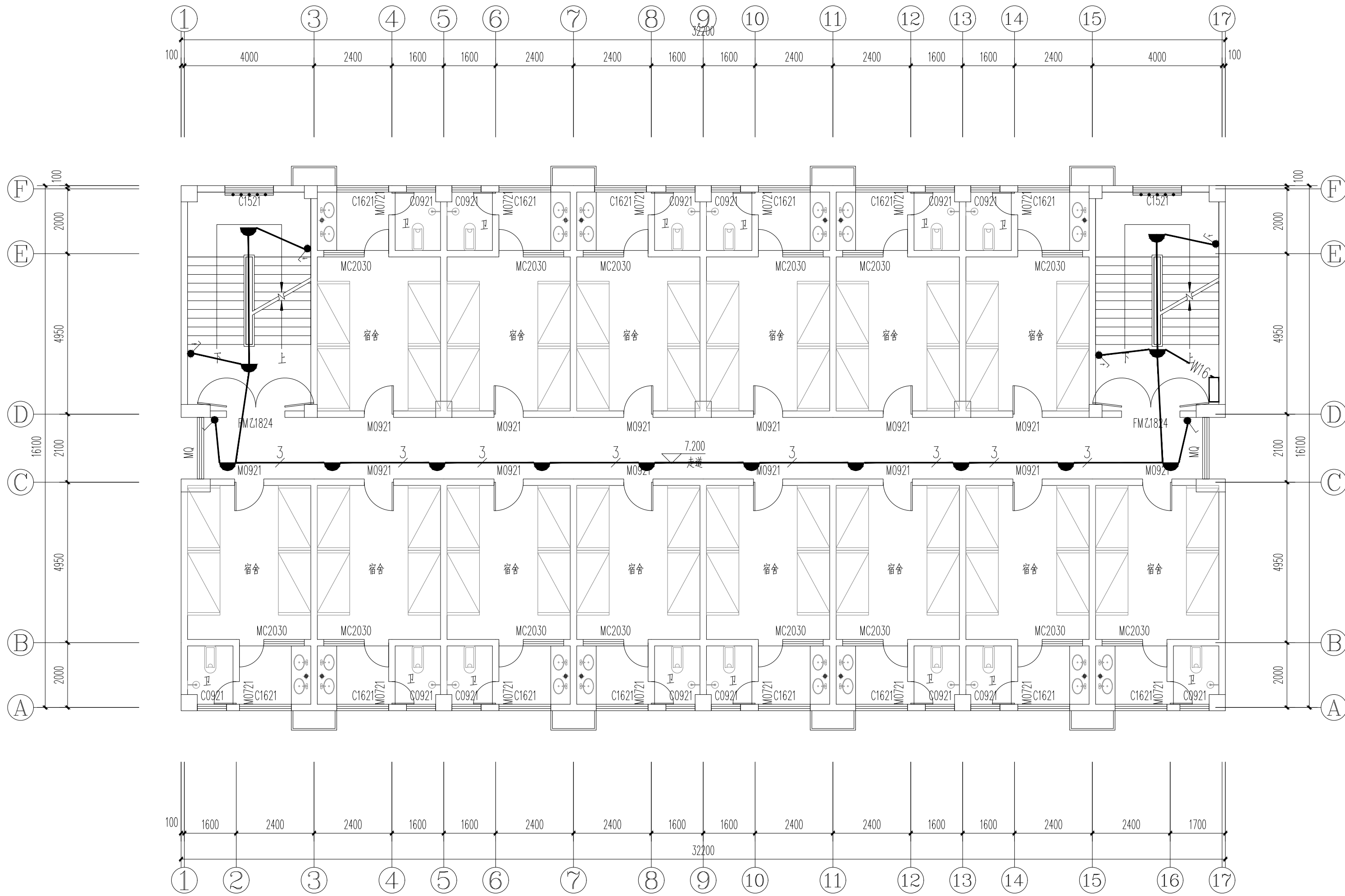
三层平面图 1:100
