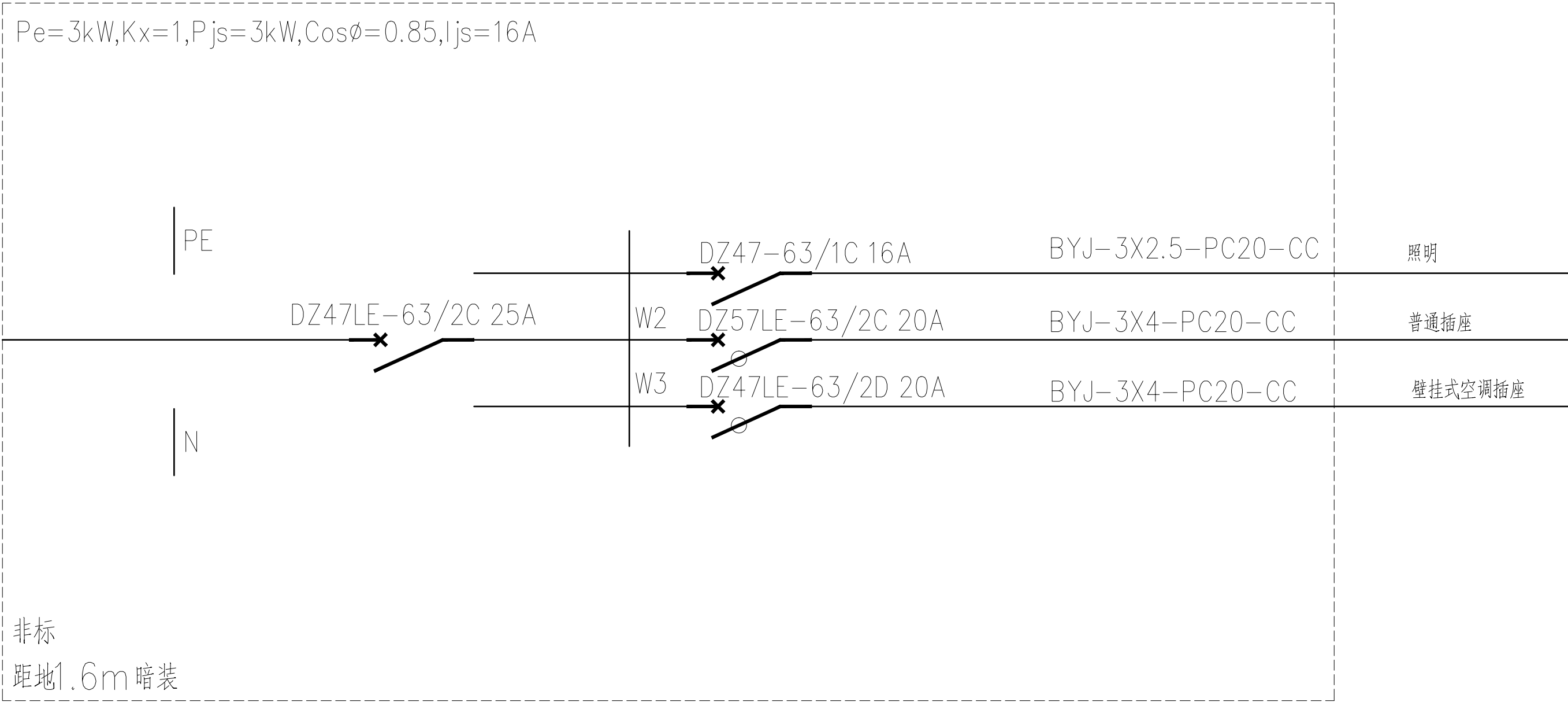
ADD1系统图
