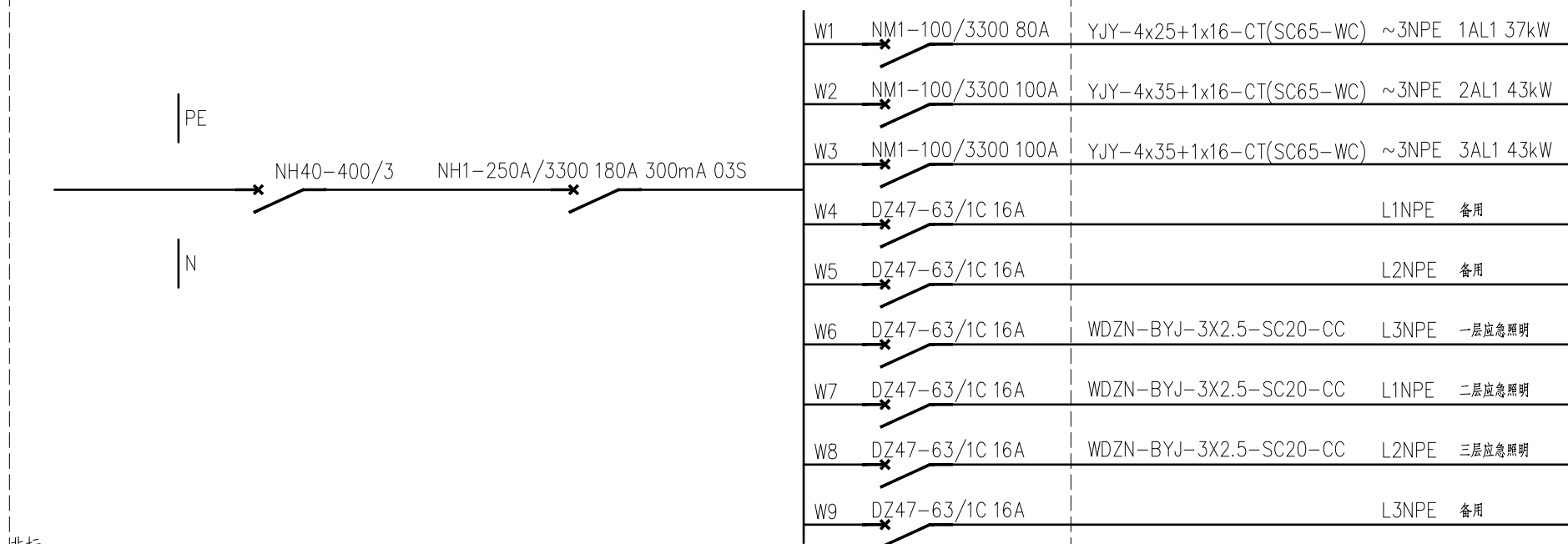
ALZ系统图
