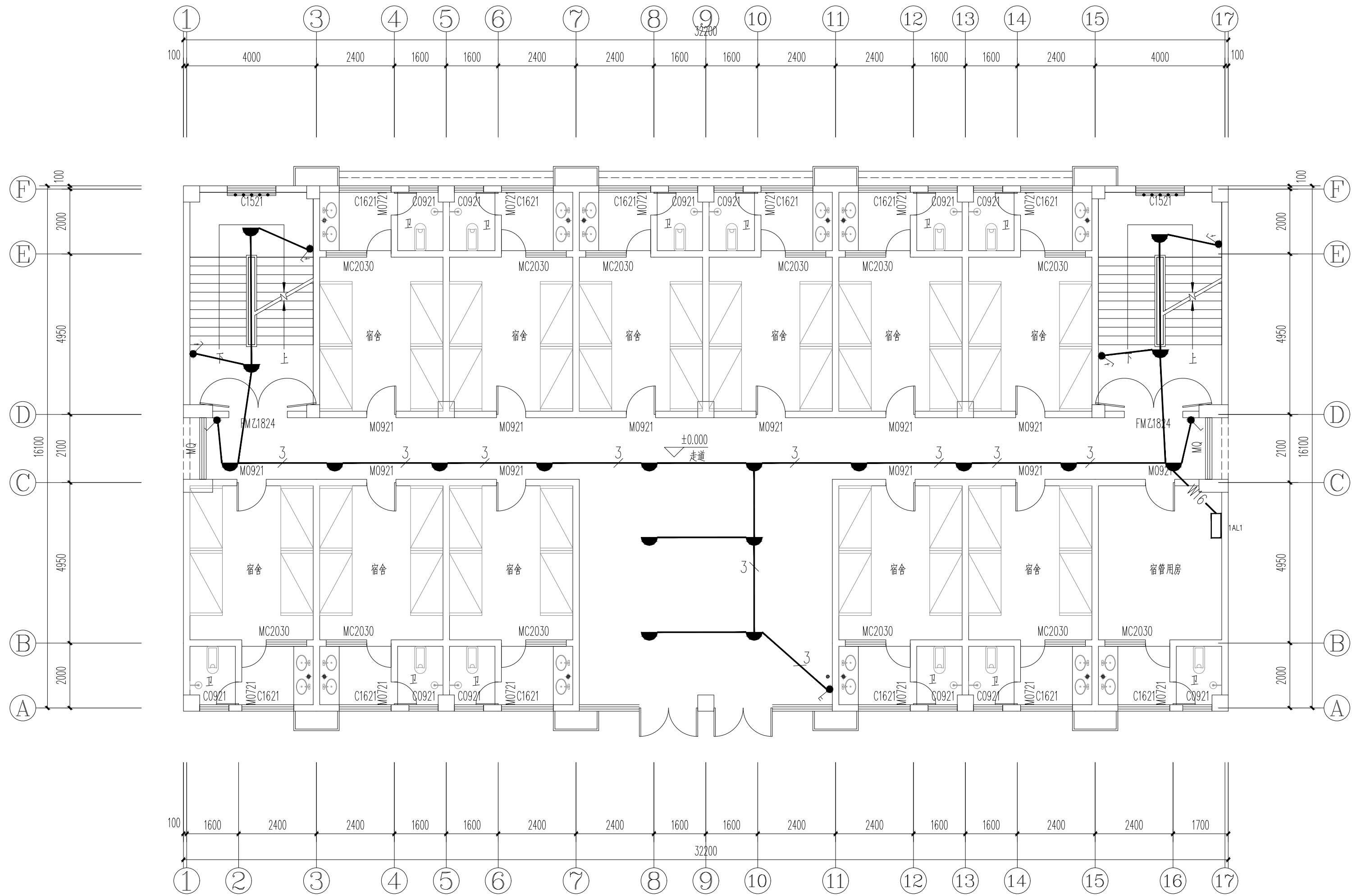
一层平面图 1:100
