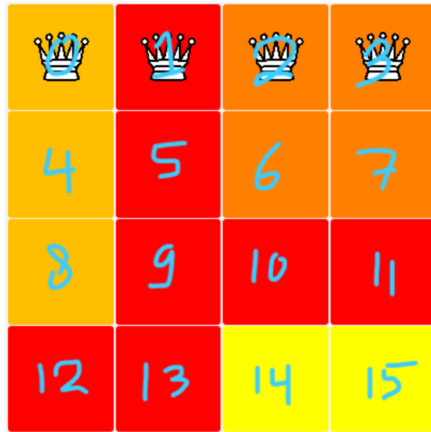
Gambar 2.1: Contoh penomoran petak pada papan berukuran 4x4
