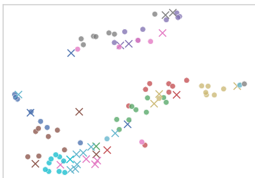
ACSF1: Temporal
