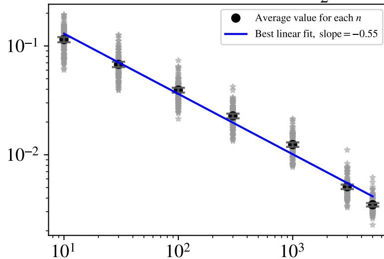
d=8 , actual slope = -\frac{2}{8}
