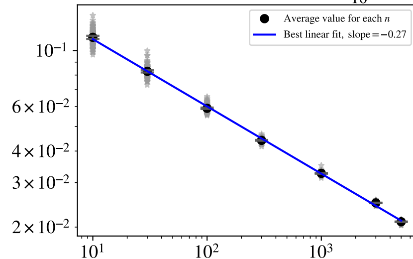
d=10 , actual slope = -\frac{2}{10}
