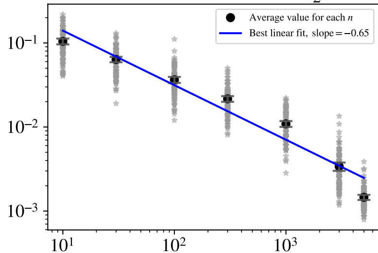
d=6 , actual slope = -\frac{2}{6}
