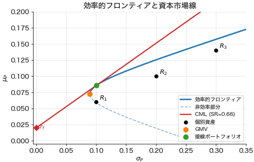
Figure 4.1: 3 資産モデルにおける効率的フロンティア（上枝の太線）、大域最小分散ポートフォリオ（GMV）、無リスク資産 r_f から引いた CML、接線ポートフォリオ。CML の傾きが最大シャープ比 SR^* となる。
