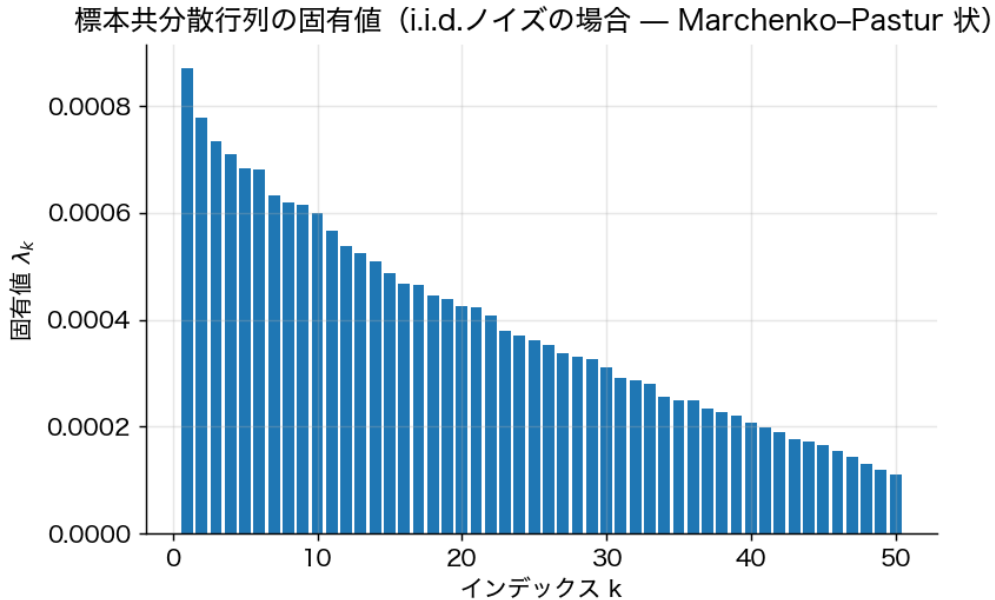
Figure 2.1: 共分散行列の固有値スペクトル例 (標本 T = 200 、 n = 50 、i.i.d. ノイズ)。最大固有値は集中・最小固有値は 0 に近く、最適化はこの「小さい固有値方向」を増幅するため推定誤差問題が深刻になる。
