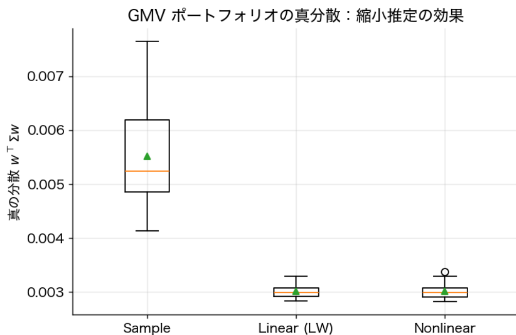
Figure 14.2: 共分散推定法の効果比較：標本共分散・線形縮小・非線形縮小それぞれを使った GMV の out-of-sample 分散。データ駆動の縮小は安定性を改善する。
