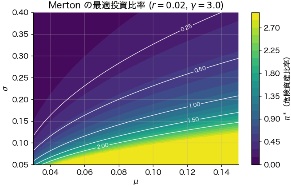
Figure 12: Merton 問題の最適投資比率 \pi^* = (\mu - r)/(\gamma\sigma^2) を (\mu, \sigma) 平面で等高線表示。ボラティリティが高いほど・期待リターンが低いほど危険資産投資を絞る。
