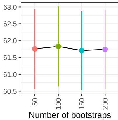
LUAD
