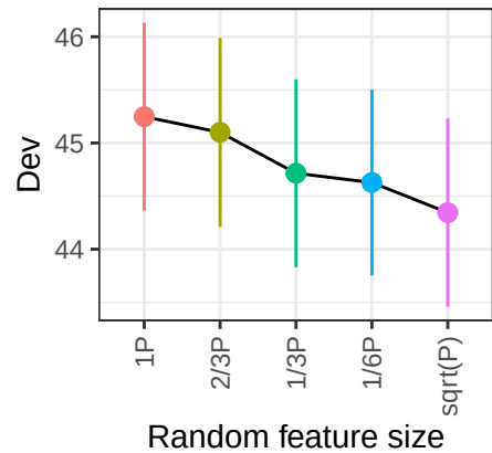
LIHC
