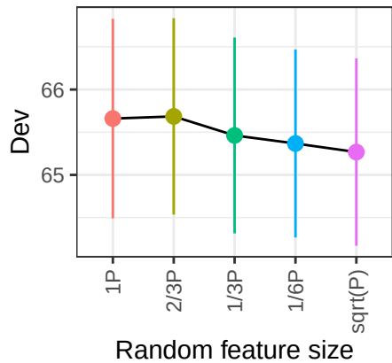
LUAD
