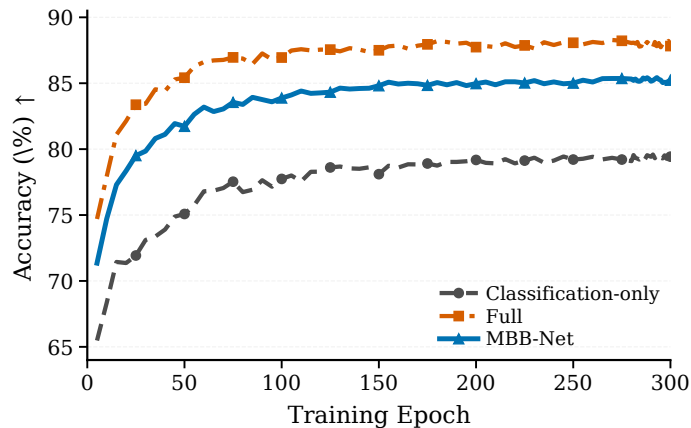
(d) ShapeNet-55: Classification Dynamics
