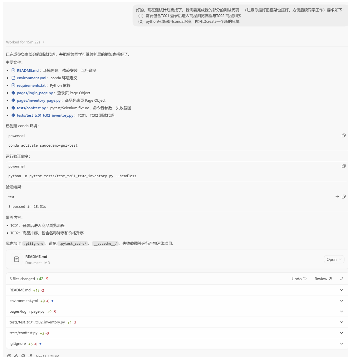
图 4：要求大模型搭建 Selenium 自动化测试框架并实现 TC01、TC02 测试脚本。
