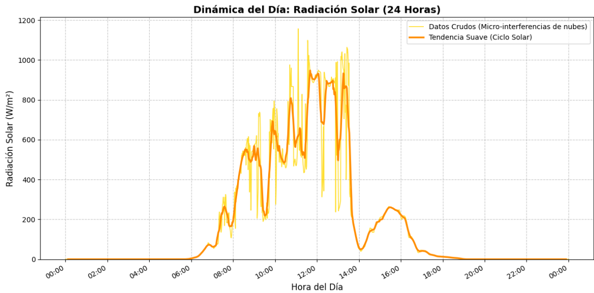
Figura 4. Ciclo diurno de Radiación Solar e Índice UV. Los patrones dentados en la lectura cruda (línea delgada) evidencian el paso transitorio de nubosidad, validados por la rápida recuperación del sensor.
