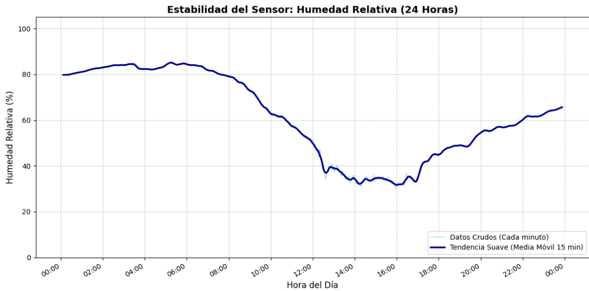
Figura 2. Comportamiento de la Humedad Relativa. Se observa el descenso o "valle" diurno natural, fundamental para calcular la ventana de secado óptima del invernadero.
