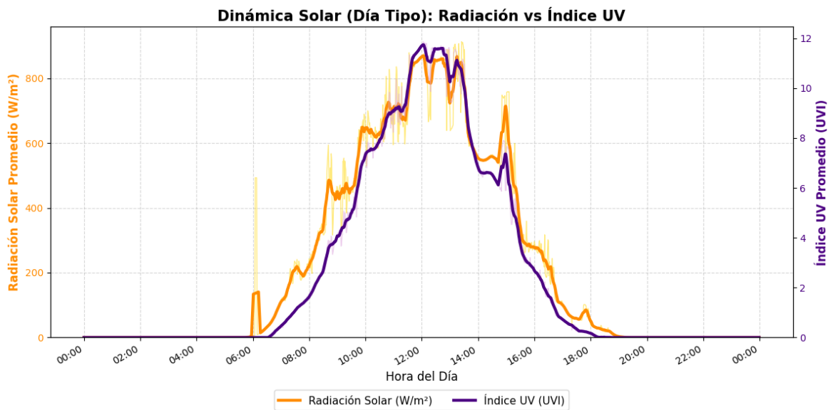
Figura 6. Relación termodinámica (radiación solar vs índice UV) utilizando el perfil base promediado de 3 días (12 al 14 de junio de 2026).
