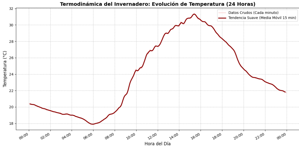
Figura 1. Evolución térmica en un ciclo de 24 horas. La línea roja gruesa representa el suavizado matemático (media móvil de 15 minutos) aplicado sobre los datos crudos para filtrar anomalías transitorias.
