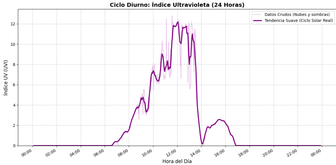
Figura 5. Dinámica Solar Combinada. Perfil base promediado de 3 días demostrando el acoplamiento perfecto entre la irradiancia máxima y el espectro UV. Nótese el aplanamiento absoluto en 0.0 durante la fase nocturna, validando la máscara de 10-bits.
