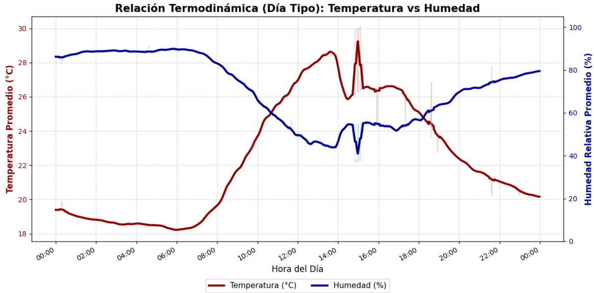
Figura 3. Relación termodinámica (Temperatura vs Humedad) utilizando el perfil base promediado de 3 días (12 al 14 de junio de 2026).
