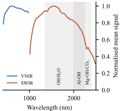
(d) Parcel mean spectrum
