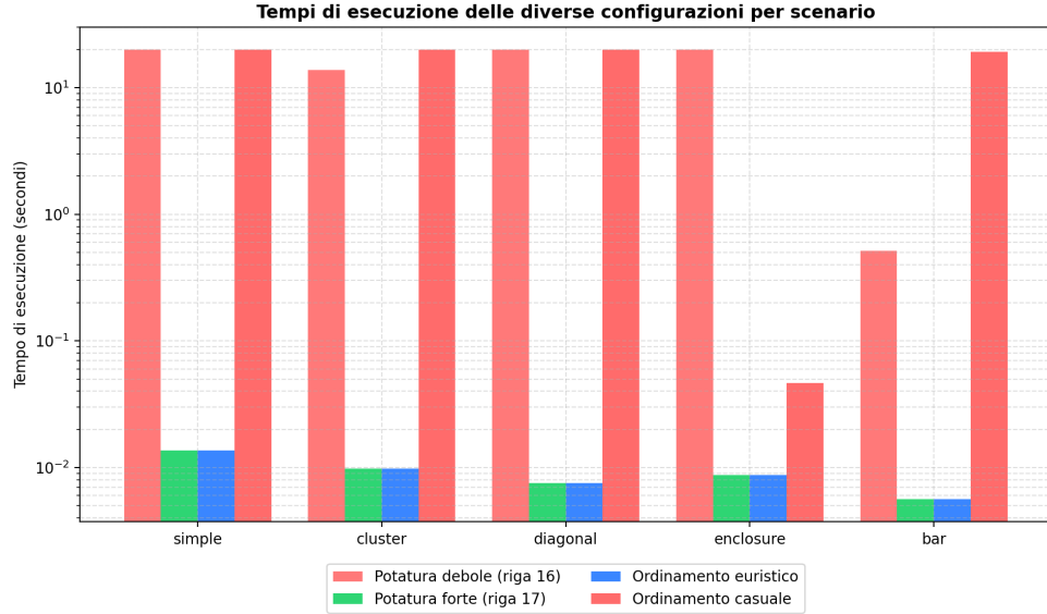
Figura 10: Tempi di esecuzione delle quattro configurazioni (potatura debole/forte, ordinamento euristico/casuale) per tipologia di ostacolo.
