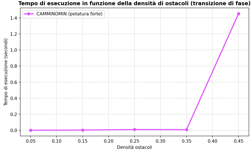
Figura 9: Tempo di esecuzione in funzione della densità di ostacoli (transizione di fase).
