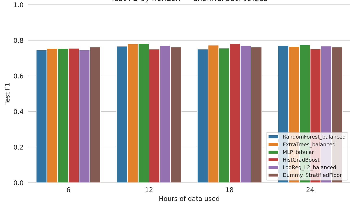
Test F1 by horizon — channel set: values
