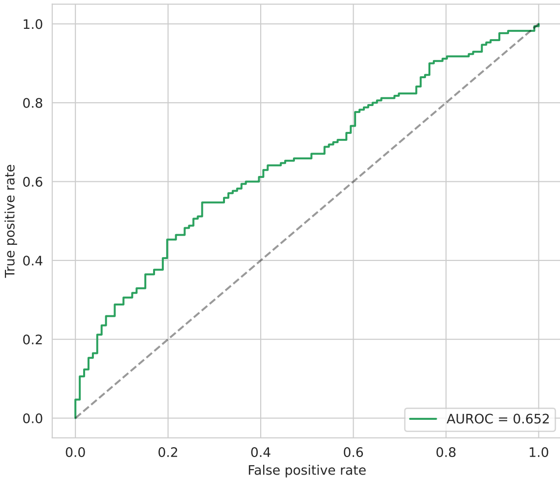
Test ROC
