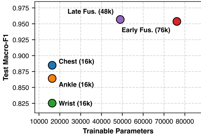
(a) Macro-F1 vs Parameters
