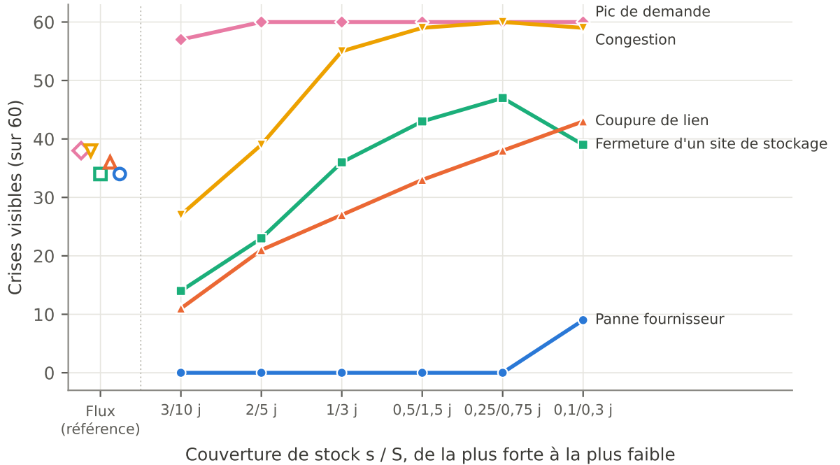
FIGURE 10 – Nombre de crises visibles sur 60 selon la couverture de stock, par nature de perturbation (réseau ISOMORPH, sans réaction). Les symboles creux, à gauche, donnent la référence de la représentation par flux.
