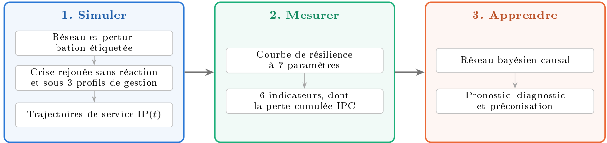
FIGURE 1 – Démarche en trois blocs. Le bloc 1 joue chaque crise sous quatre politiques de gestion ; le bloc 2 résume chaque trajectoire par une courbe à sept paramètres et six indicateurs ; le bloc 3 apprend un réseau bayésien dont la structure respecte l'ordre temporel d'une crise, et en tire pronostic, diagnostic et préconisation.
