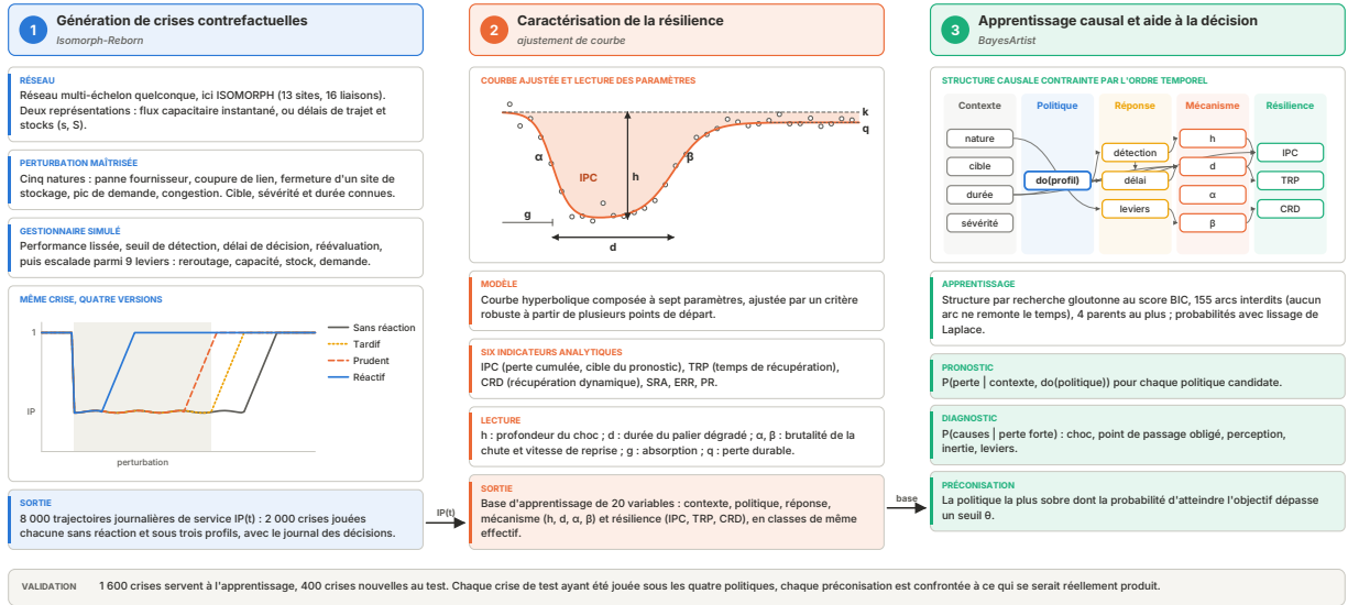
Figure 1: Démarche en trois blocs. Le bloc 1 joue chaque crise sous quatre politiques de gestion ; le bloc 2 résume chaque trajectoire par une courbe à sept paramètres et six indicateurs ; le bloc 3 apprend un réseau bayésien dont la structure respecte l'ordre temporel d'une crise, et en tire pronostic, diagnostic et préconisation.
