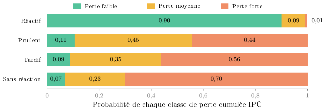
FIGURE S3 – Pronostic de la perte cumulée selon la politique, pour la fermeture longue d’un site situé sur un point de passage obligé : distribution des trois classes d’IPC inférée par le réseau appris.
