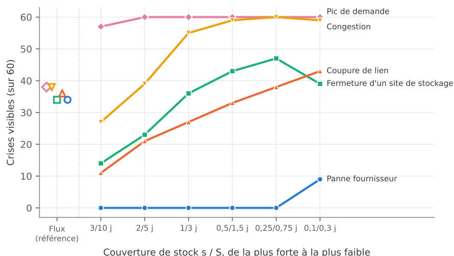
FIGURE S4 – Nombre de crises visibles sur 60 selon la couverture de stock, par nature de perturbation (réseau ISOMORPH, sans réaction). Les symboles creux, à gauche, donnent la référence de la représentation par flux.
