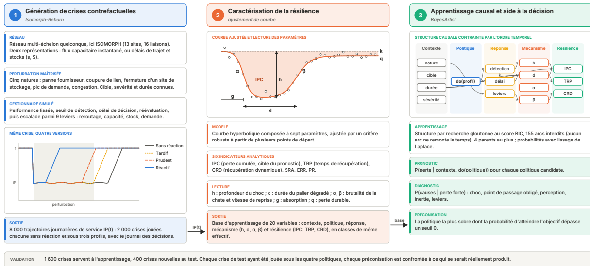
FIGURE S5 – Démarche détaillée en trois blocs : entrées, traitements et sorties de chaque bloc.
