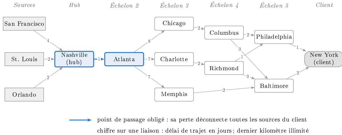
FIGURE S3 – Réseau ISOMORPH d'origine représenté par échelons, des trois sources au client.
