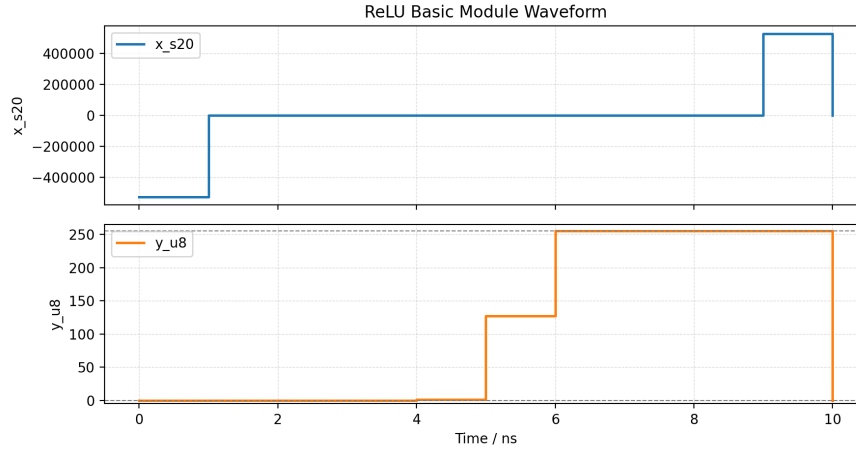
图 1: 基础模块波形: relu_s20 的截断与饱和行为
