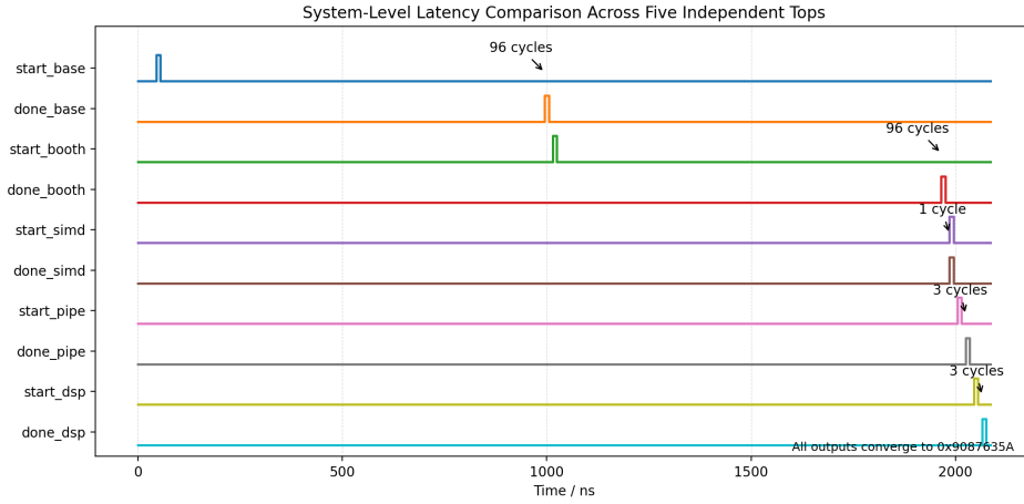
图 2: 系统级波形: 5 个独立顶层的 start/done 延迟对比
