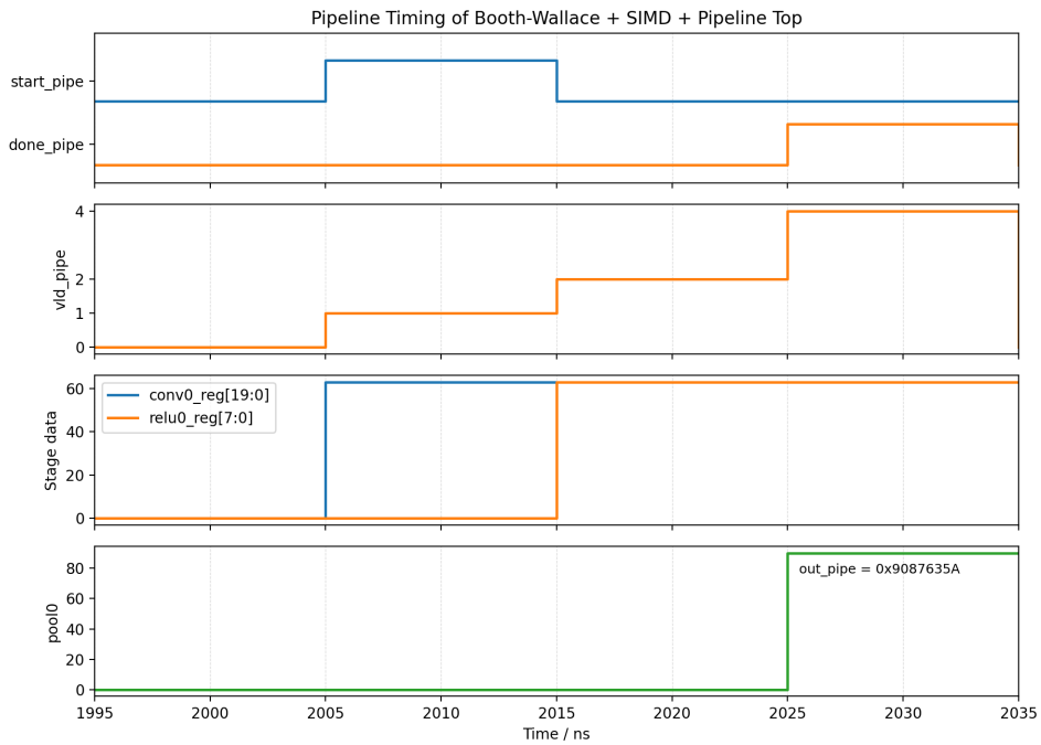
图 3: 流水线波形: 卷积寄存、ReLU 寄存与输出寄存的三级推进
