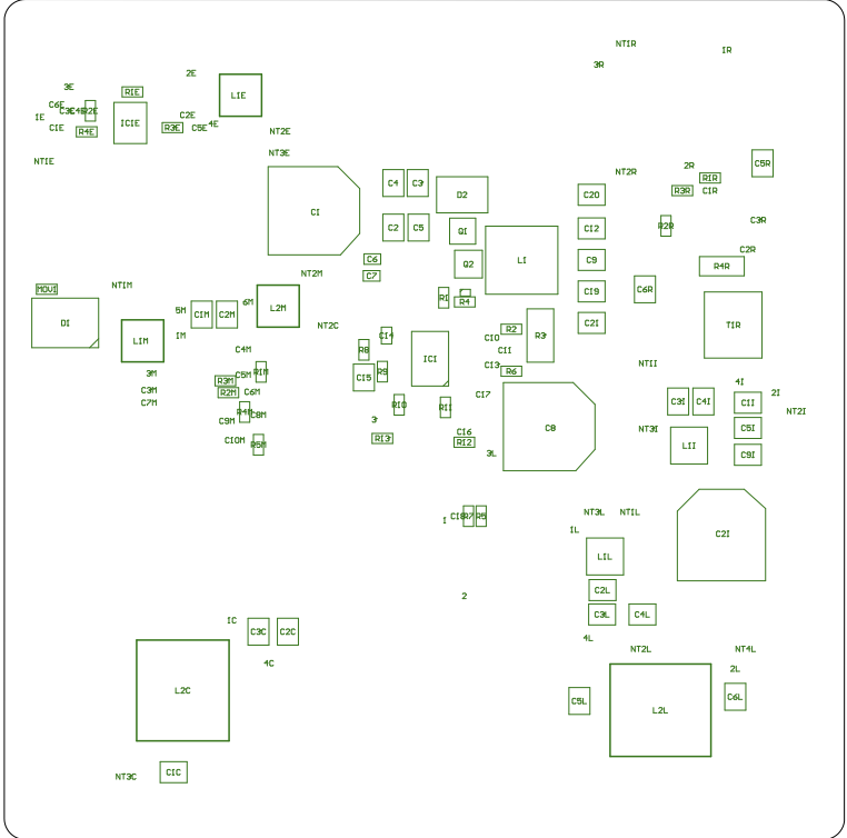
TOP (Scale 1:1)
