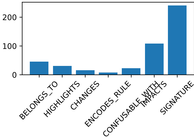
Edge types
